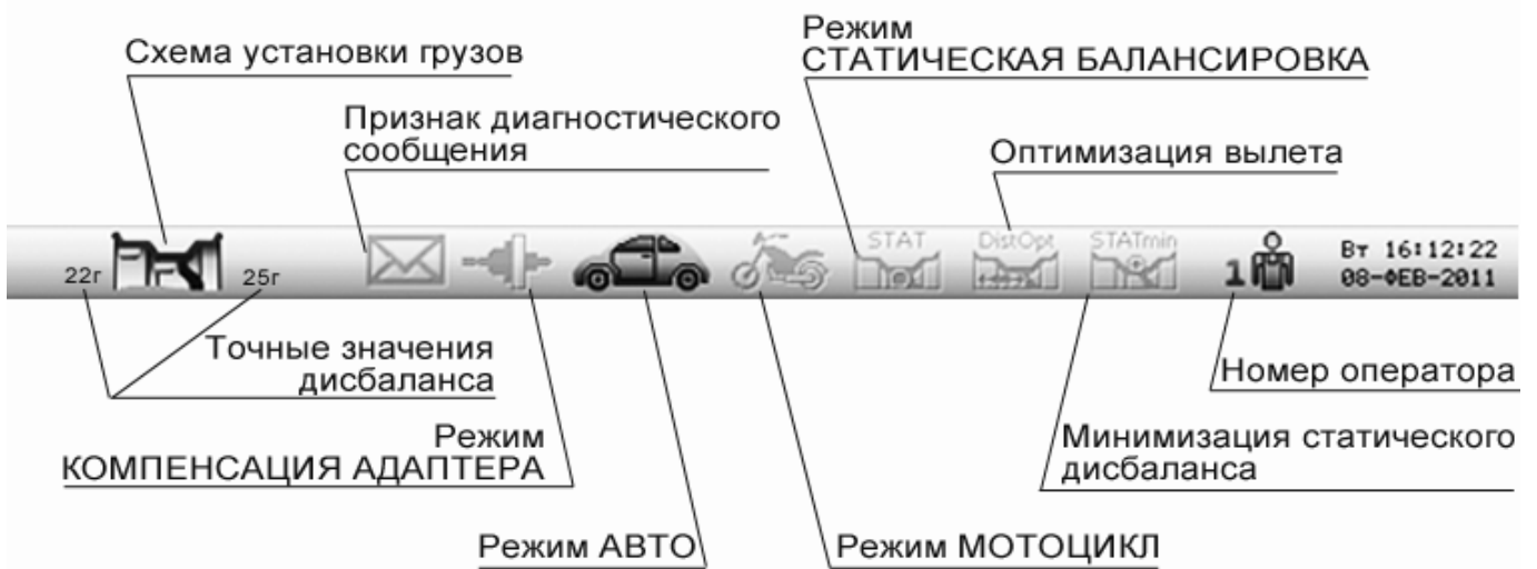
Рисунок 4.5 – Информационное поле
