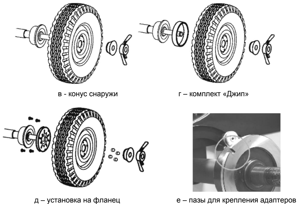
Рисунок 5.1 – Установка колеса
