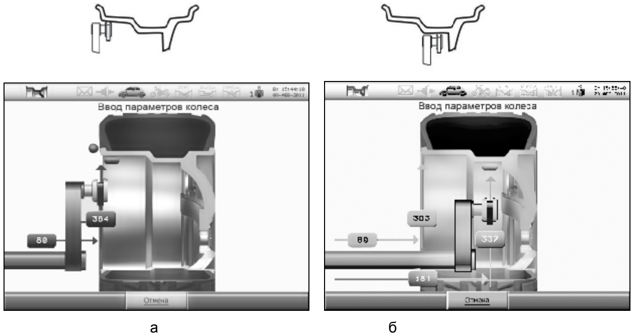
Рисунок 6.10 – Ввод размеров
