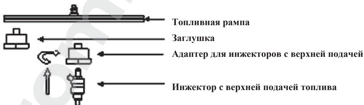
Рис. 2.1 Установка адаптера инжектора с верхней подачей топлива
